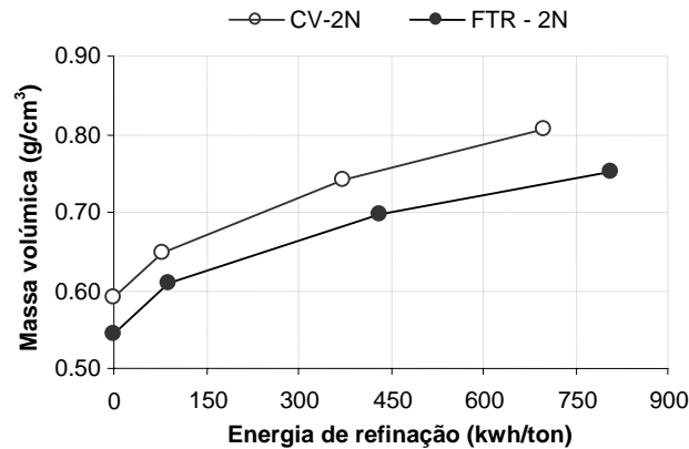
Figura 2 - Evolução da massa volúmica das folhas em função da energia de refinação
