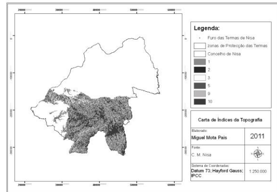
Fig. 4 – Carta de índices da topografia (T)
