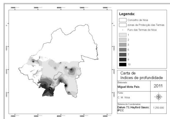
Fig. 2 – Carta interpolada para o atributo profundidade (D)
