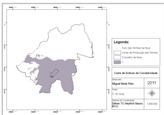
Fig. 5 – Carta de índices da condutividade Hidráulica (C)
