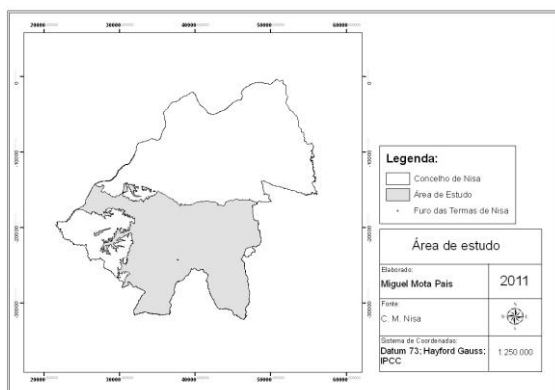
Fig. 1 – Área de estudo delimitada para aplicação vulnerabilidade “DRASTIC”
