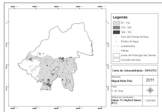
Fig. 6 – Carta de vulnerabilidade DRASTIC
