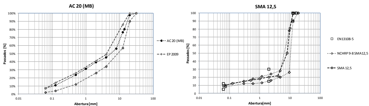
Figura 1: Curvas granulométricas das misturas AC20 e SMA 12,5
