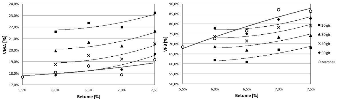
Figura 8: Evolução do VMA e do VFB com a percentagem em betume para a mistura SMA 12,5
