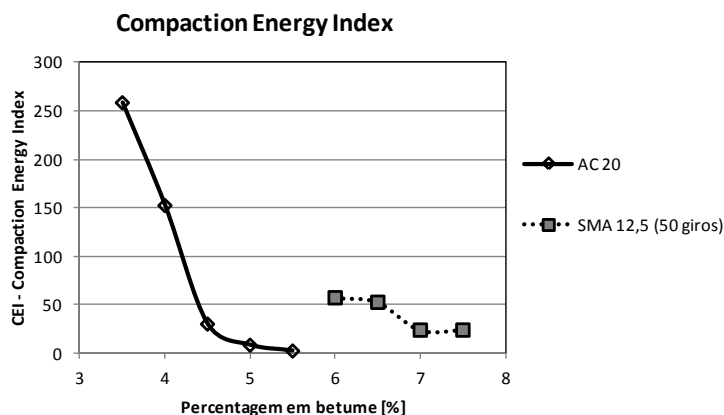
Figura 10: Variação do CEI com a porcentagem em betume
