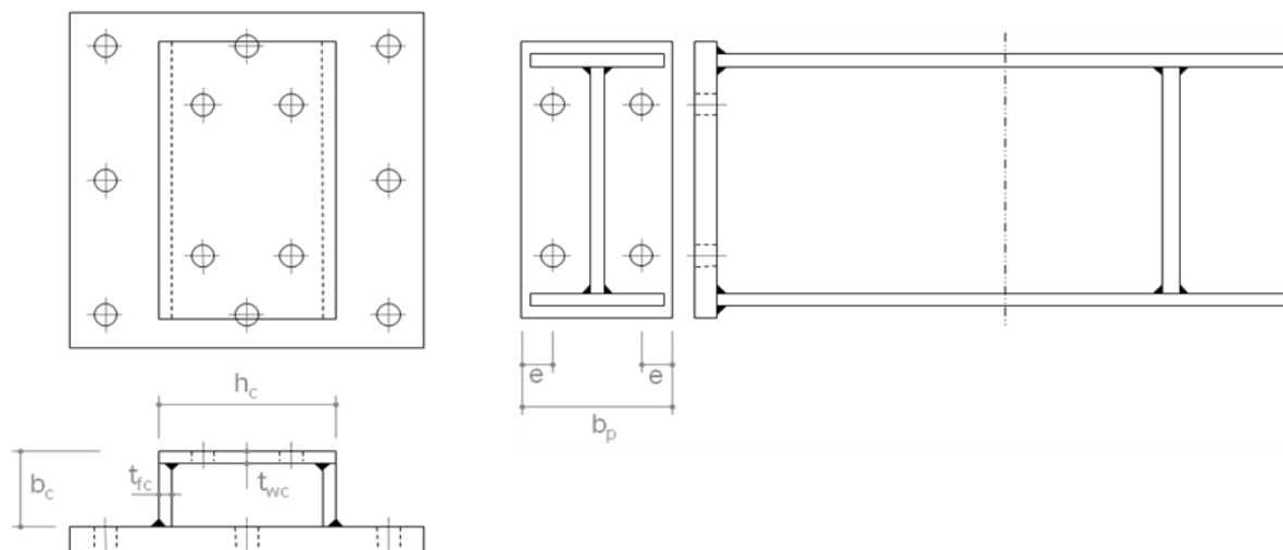
Figura 2. Esquema do protótipo e da viga.
