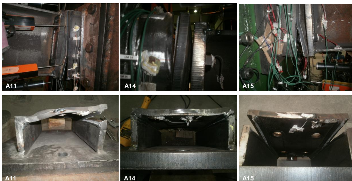
Figura 12a. Rotura dos cordões de soldadura nos protótipos A-11, A-14 e A-15.
