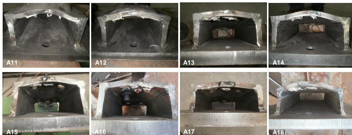
Figura 8. Deformação na zona superior dos protótipos nos ensaios monotónicos.
