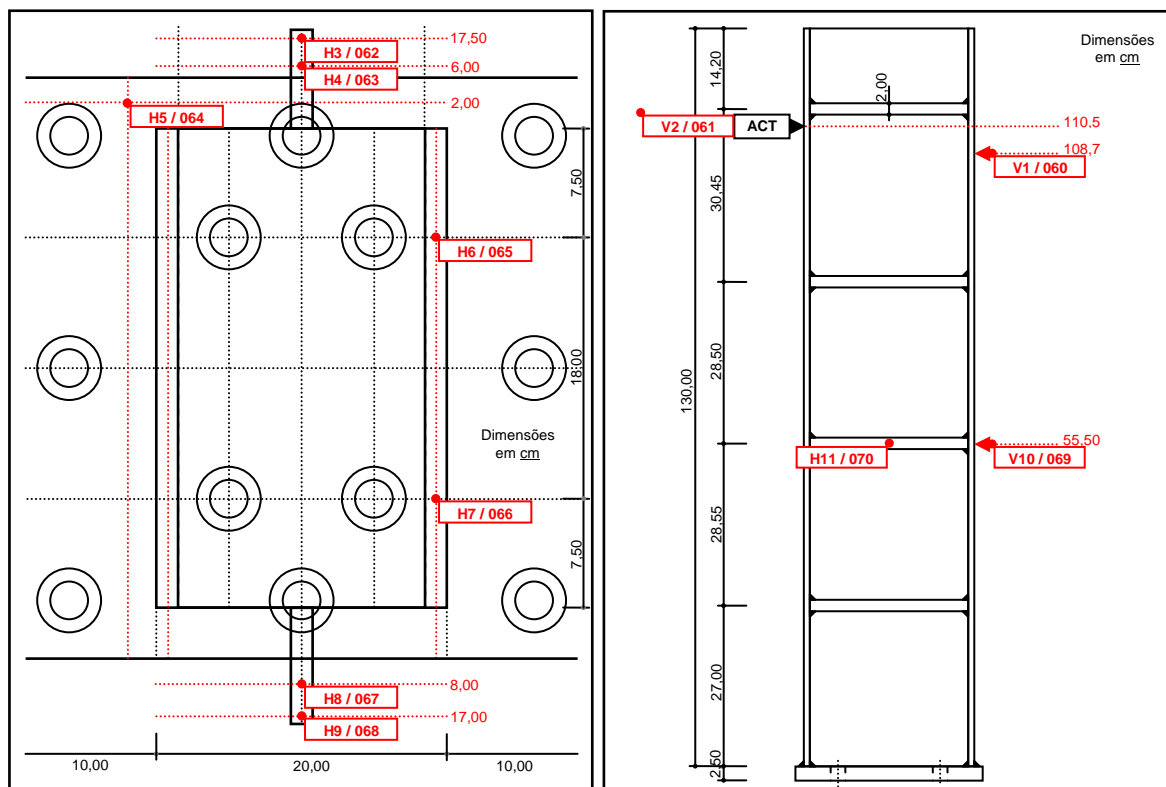
Figura 4. Esquema de colocação dos defletómetros (à esquerda no perfil em U e à direita na viga).
