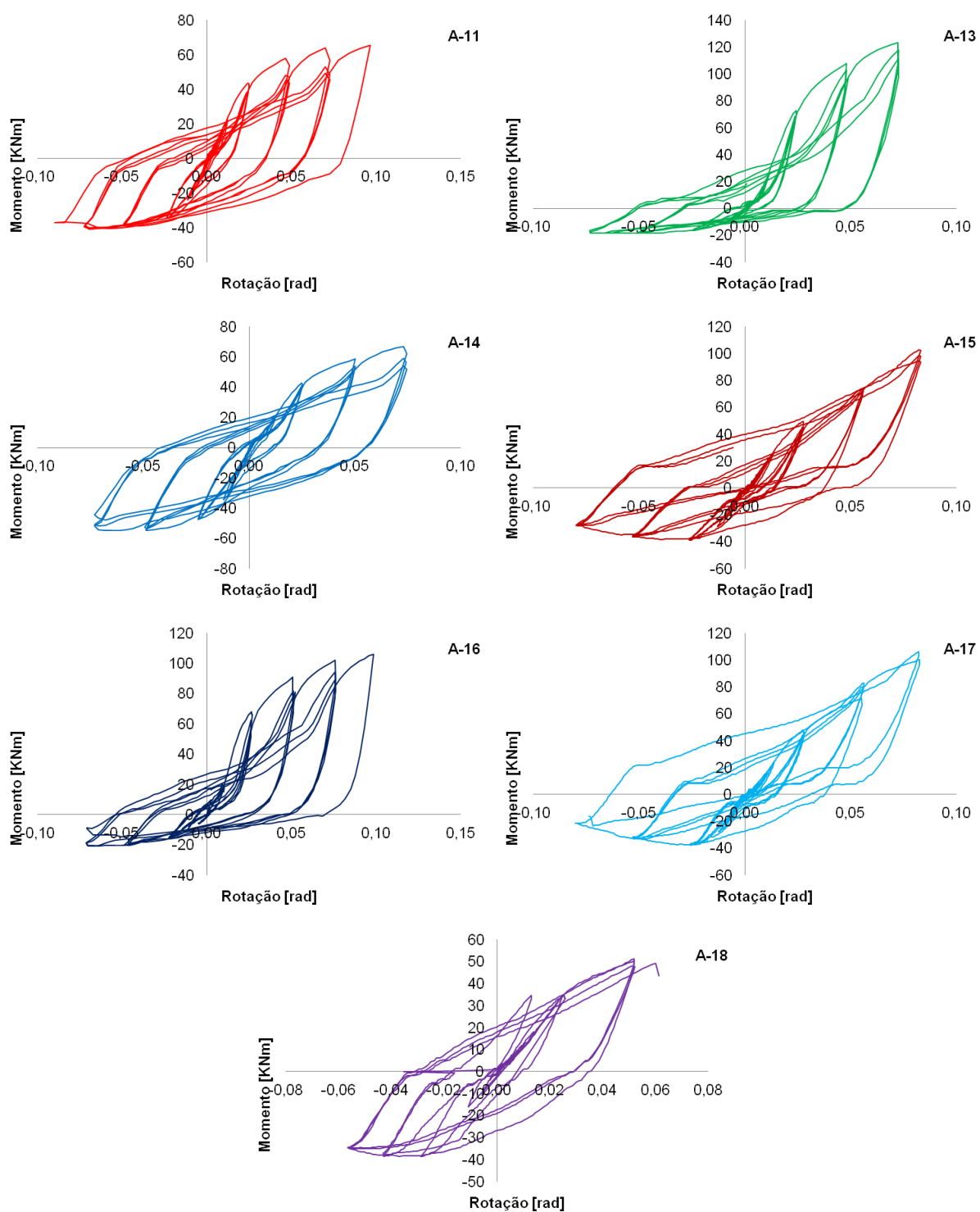
Figura 15. Diagramas de curvas histeréticas momento-rotação.
