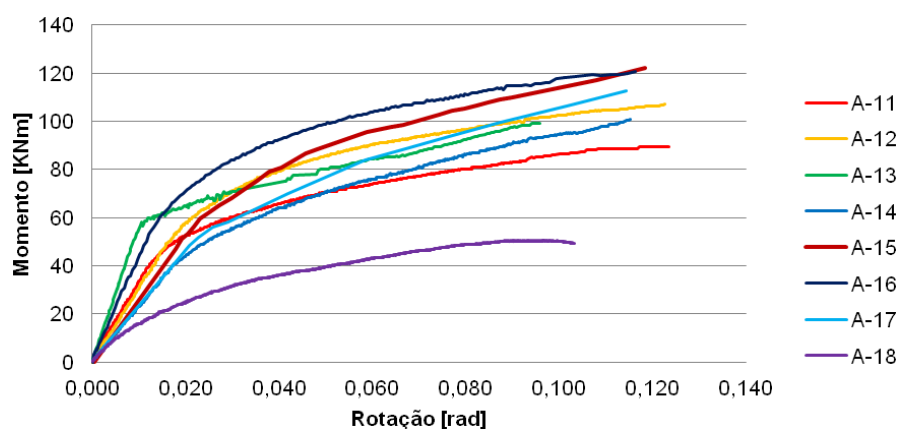
Figura 10. Diagramas momento-rotação para os ensaios monotónicos.
