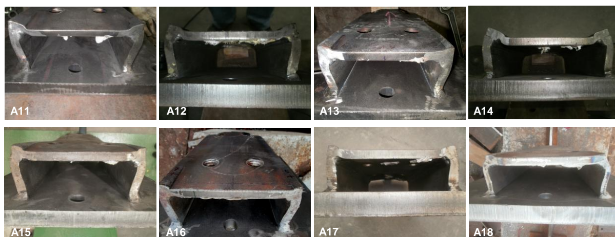
Figura 9. Deformação na zona inferior dos protótipos nos ensaios monotónicos.
