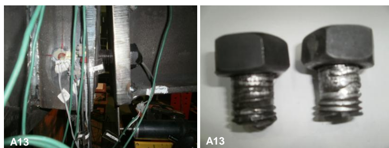
Figura 14. Detalhes do escorregamento dos parafusos na ligação A-13.
