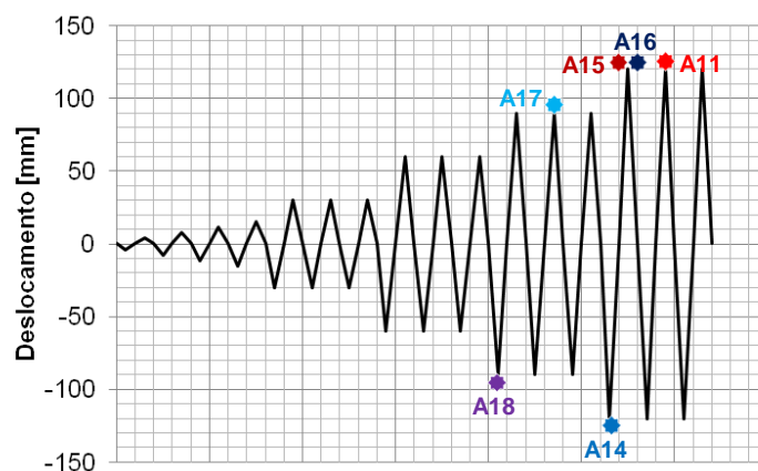
Figura 11. Localização da rotura da ligação para cada um dos ensaios cíclicos.
