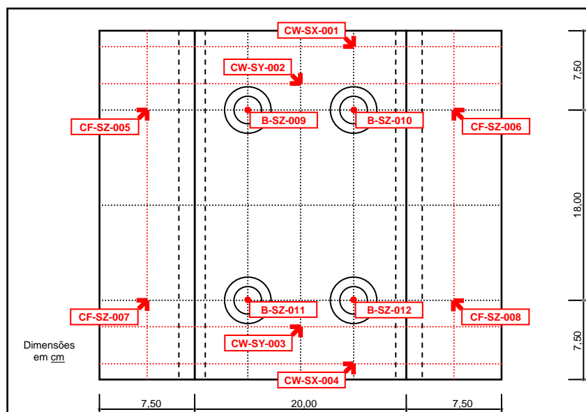
Figura 5. Esquema de colocações dos extensómetros.
