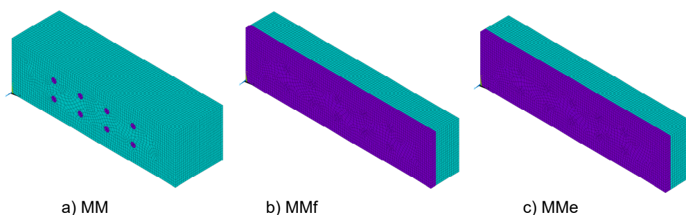
Figura 3: Malhas. a) ligação madeira-madeira MM; b) ligação madeira-chapa fina MMf; c) ligação madeira-chapa espessa MMe
