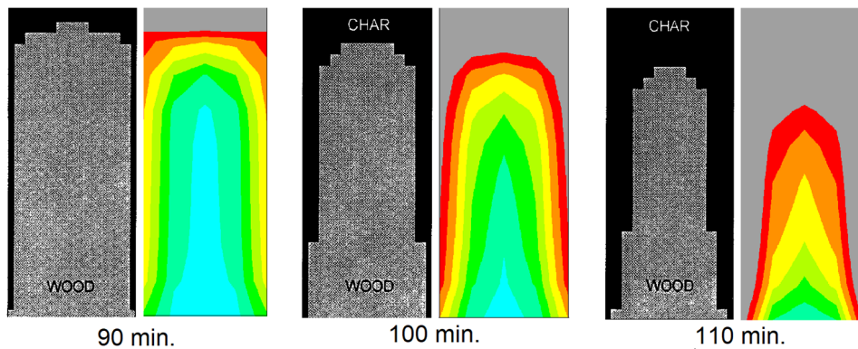
Figura 5: Comparação da evolução da carbonização com o modelo M3
