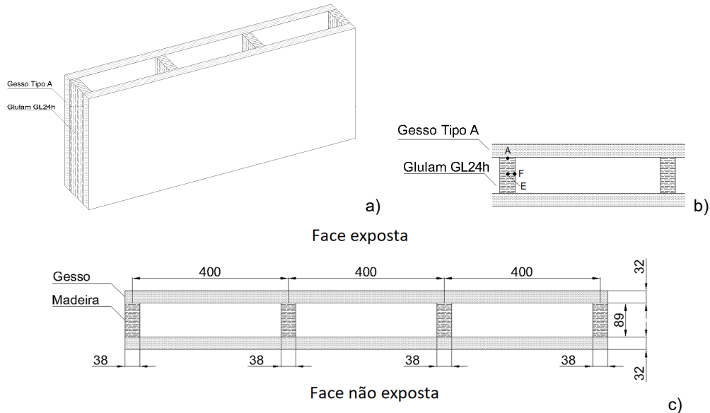
Figura 1: a) Modelo construtivo, b) Pontos de medição; c) Dimensões
