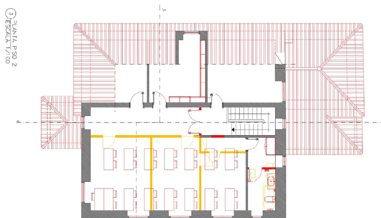
Figura 3: Planta do piso 1
