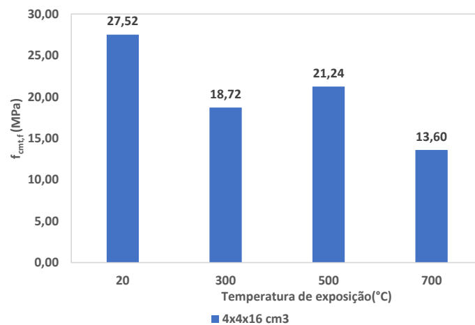
Figura 6 – Resultados do ensaio de resistência à tração por flexão.
