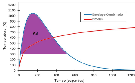
a) Área equivalente no envelope de fogos em árvores e arbustos.
