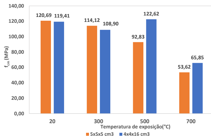
Figura 5 – Resistência à compressão após exposição a temperaturas elevadas.
