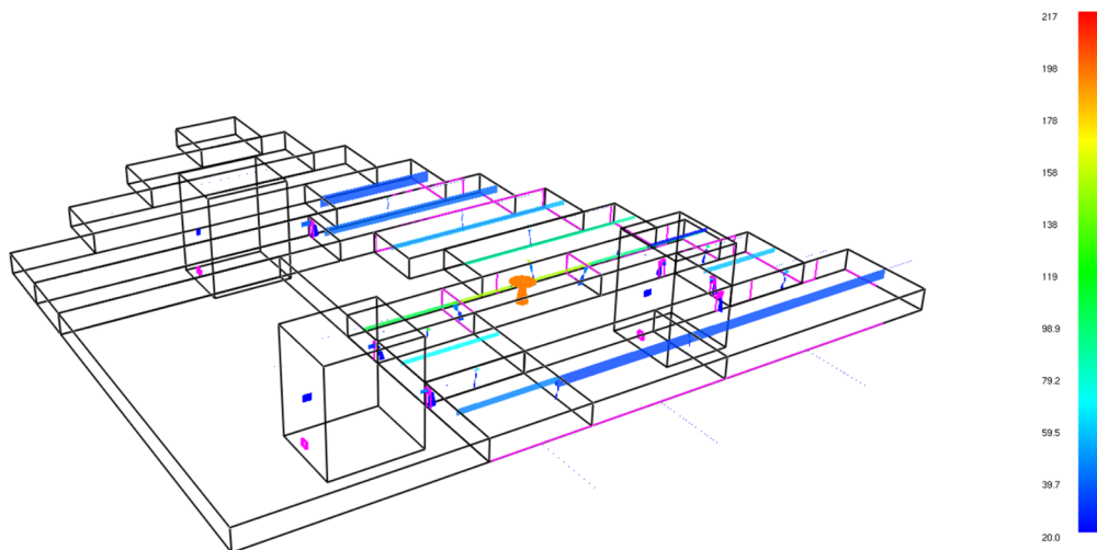
Figura 2: Imagem da simulação do CFAST, mostrando-se uma visualização 3D da altura da camada de fumo e respetiva temperatura
