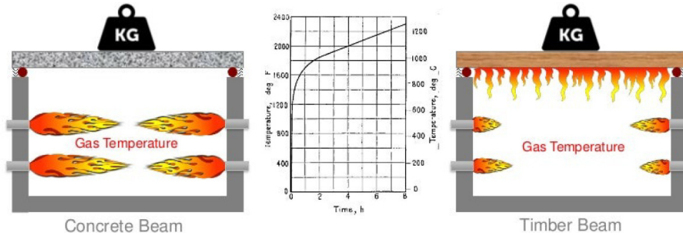
Figura 1: Teste laboratorial de incêndio em forno com curva ISO-834. Diferenças entre elementos estruturais combustíveis e não combustíveis.
