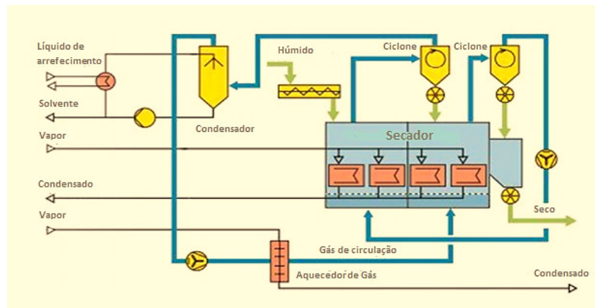
Figura 3 - Esquema de secador industrial por recirculação de calor
