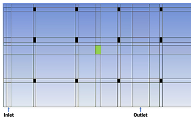
Figura 2: Esquema 2D da geometria do parque de estacionamento, com identificação das zonas de insuflação e de extração, assim como a localização do ventilador de indução (marcado a verde)
