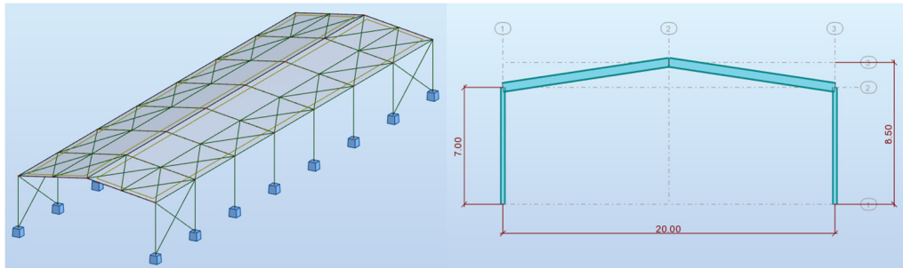
Figura 4: Estrutura da nave industrial dimensionada no ARSA; Geometria do pórtico tipo da estrutura, representação do contraventamento e definição do sistema de contraventamento
