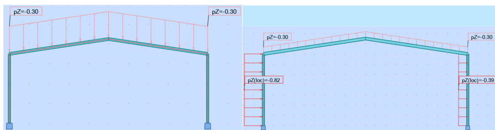
Figura 5: Carga de fogo sobre o pórtico 1 para as combinações para as ações de sobrecarga e do vento como ações variáveis de base.
