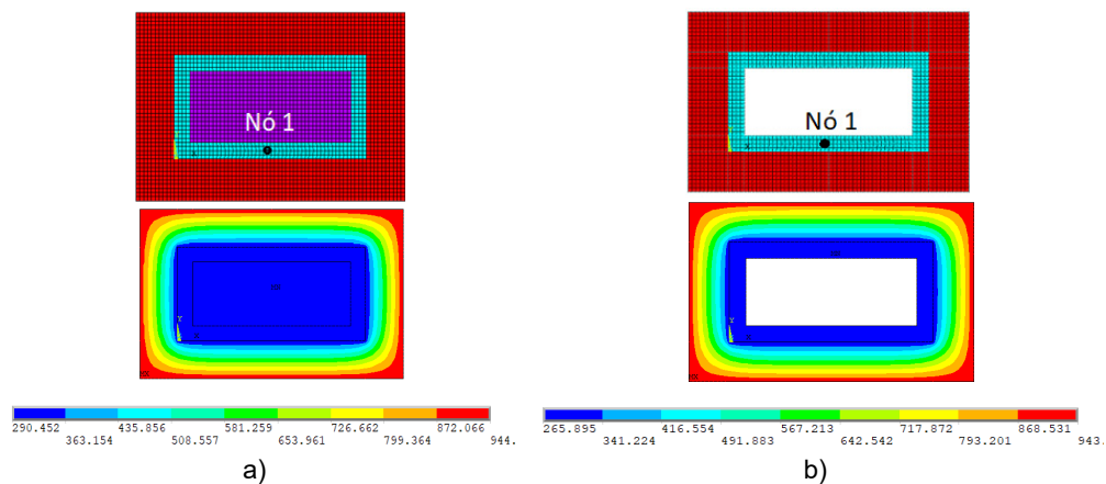
Figura 6: Temperatura dos perfis protegidos aos 3600 segundos de exposição.
