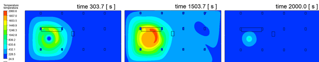
Figura 7: Contornos da temperatura ao longo do tempo no segundo incêndio
