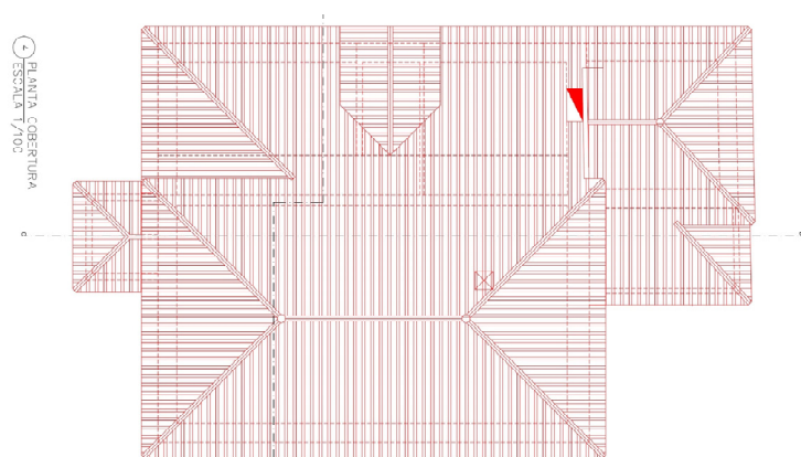
Figura 5: Planta da cobertura
