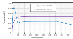
Figura 15: Cenário c) curva de acumulação de faúlhas + curva envelope de fogos em árvores e arbustos & curva de fogo exterior na fachada de habitação.
