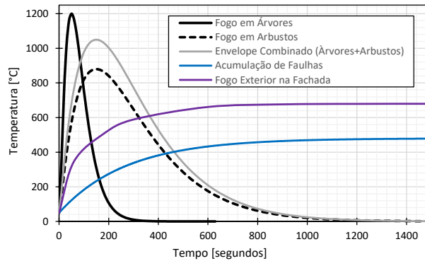
Figura 8: Curvas usadas para a simulação da ação do fogo florestal numa habitação.
