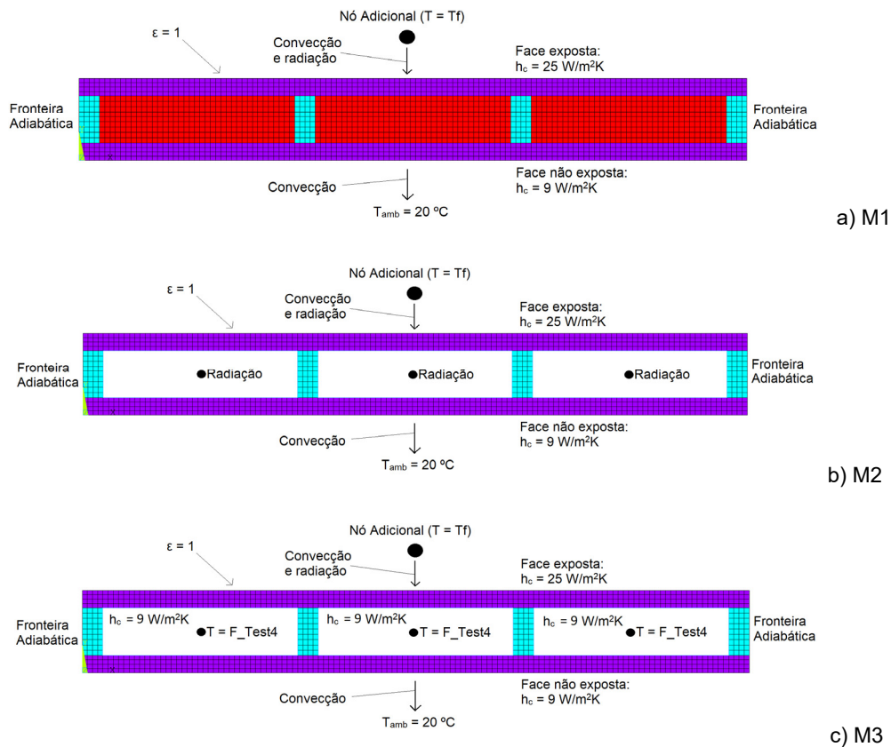
Figura 2: Malhas e condições de fronteira.
