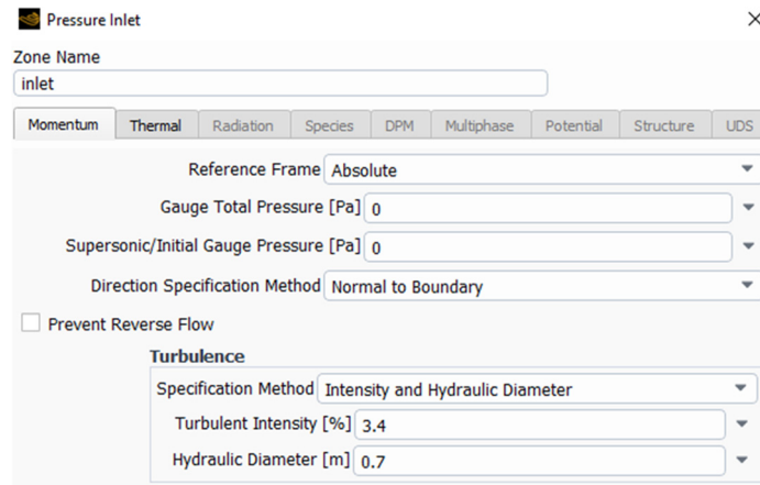
Figura 3: Definição da condição de fronteira de entrada ( inlet )
