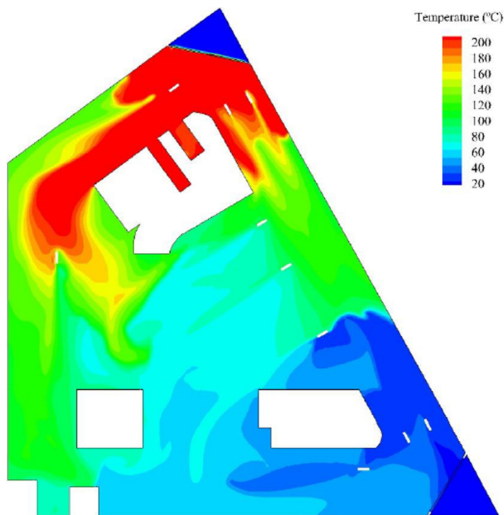
Figura 1: Imagem da simulação CFD, mostrando-se a temperatura dos gases a 2 m do chão, decorridos 20 minutos de incêndio
