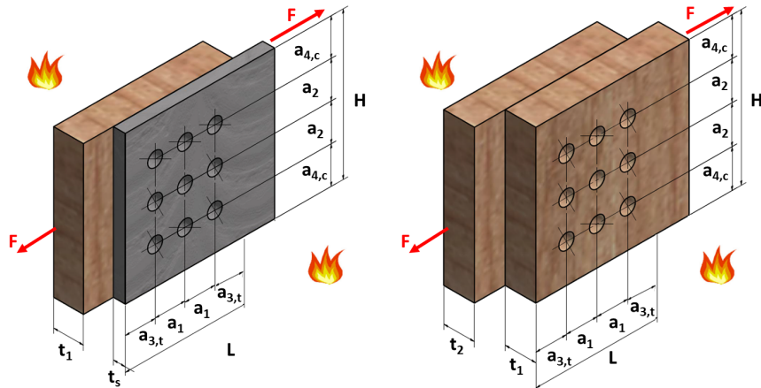
Figura 1: Modelos de ligação madeira-aço (esquerda) e madeira-madeira (direita)
