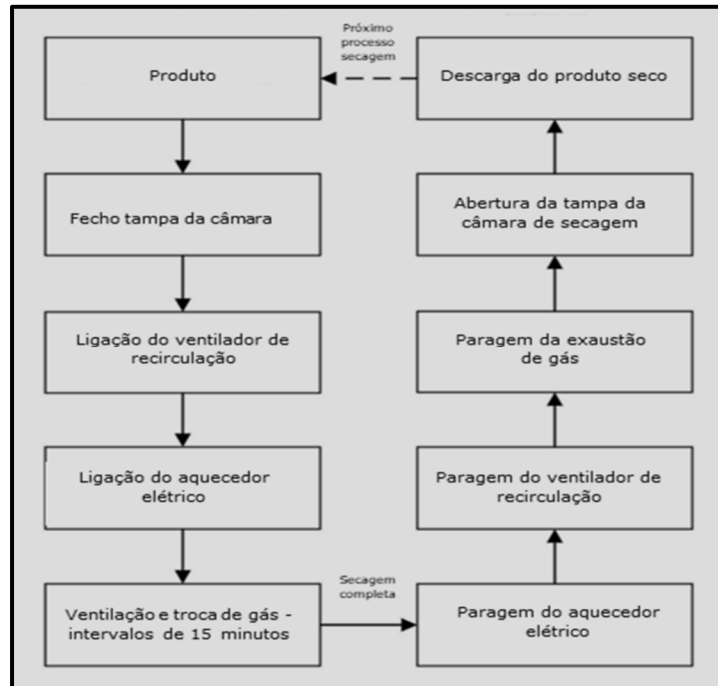
Figura 4 – Ciclo de operações básicas do processo de secagem
