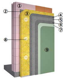
Figura 4: Solução ETIC anti-fogo para a fachada das paredes.
