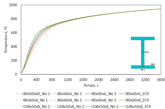
Figura 5: Temperatura dos perfis I. Comparação entre o método numérico e o Método Simplificado do Eurocódigo 9 Parte 1-2
