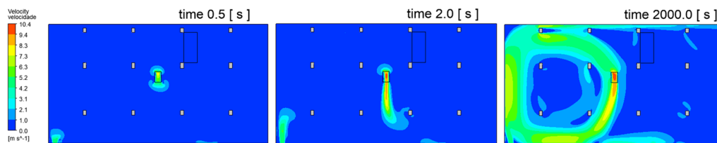
Figura 5: Contornos da velocidade ao longo do tempo
