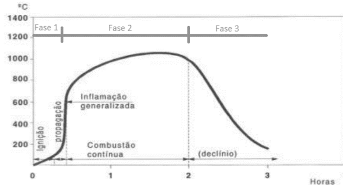
Figura 2: Curva de Fogo Natural.
