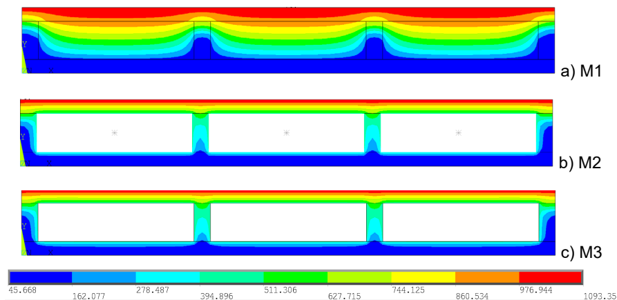
Figura 4: Campo de temperaturas para o instante final de exposição.
