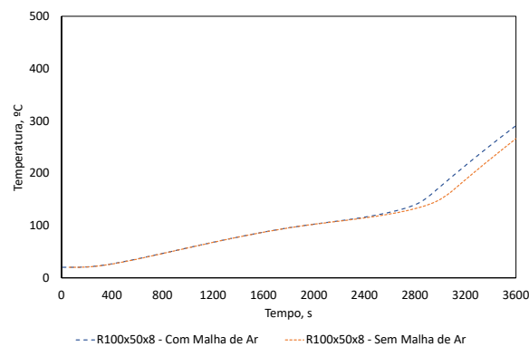
Figura 7: Temperatura do perfil retangular protegido
