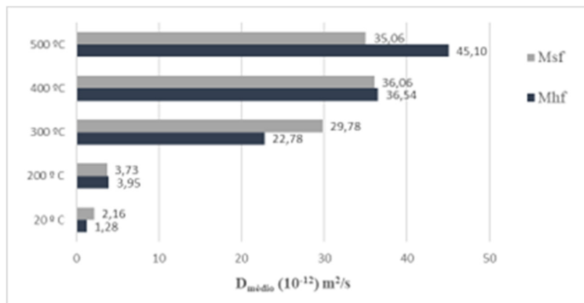
Figura 5 - Coeficiente de migração dos cloretos aos 28 dias de idade, considerando a variação do tipo de fibras.
