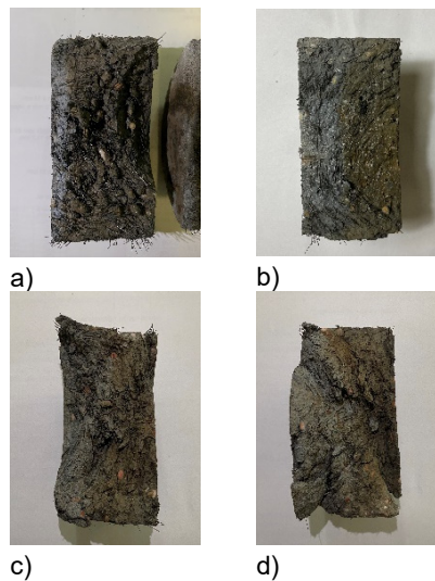
Figura 4 - Provetes de ensaio à migração de cloretos em regime não-estacionário: a) após exposição a 200°C; b) após exposição a 300°C; c) após exposição a 400°C; d) após exposição a 500°C.
