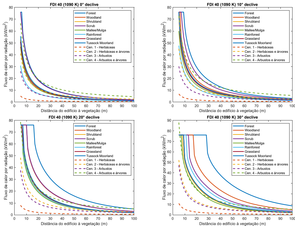
Figura 2: Fluxo de radiação térmica incidente para diferentes declives do terreno – Linhas cheias: AS3959:2018; linhas a tracejado D8591/2022 para APPS
