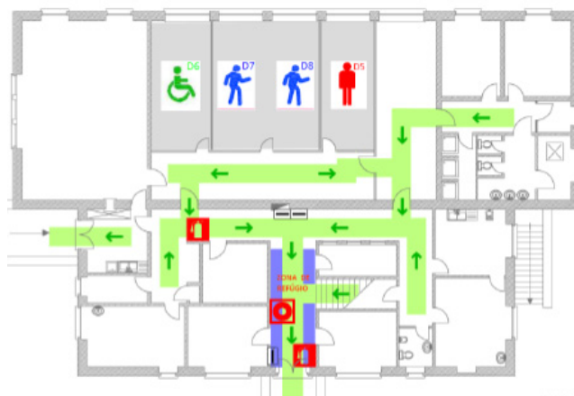
Figura 3 – Localização dos pacientes (D5, D6, D7, D8) e caminhos de evacuação no piso térreo
