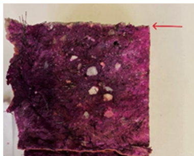
Figura 6 - Provetes de ensaio à carbonatação acelerada, frente profundidade de carbonatação.
