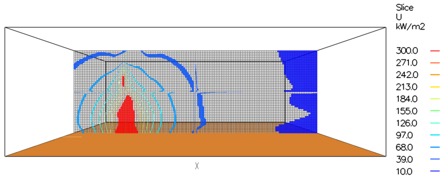
Figura 3: Intensidade de radiação integrada em todas as direções, n_{\theta} = 800
