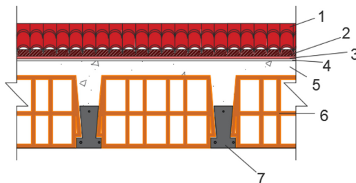
Figura 5: Solução de telha cerâmica com isolamento de Rockwool.
