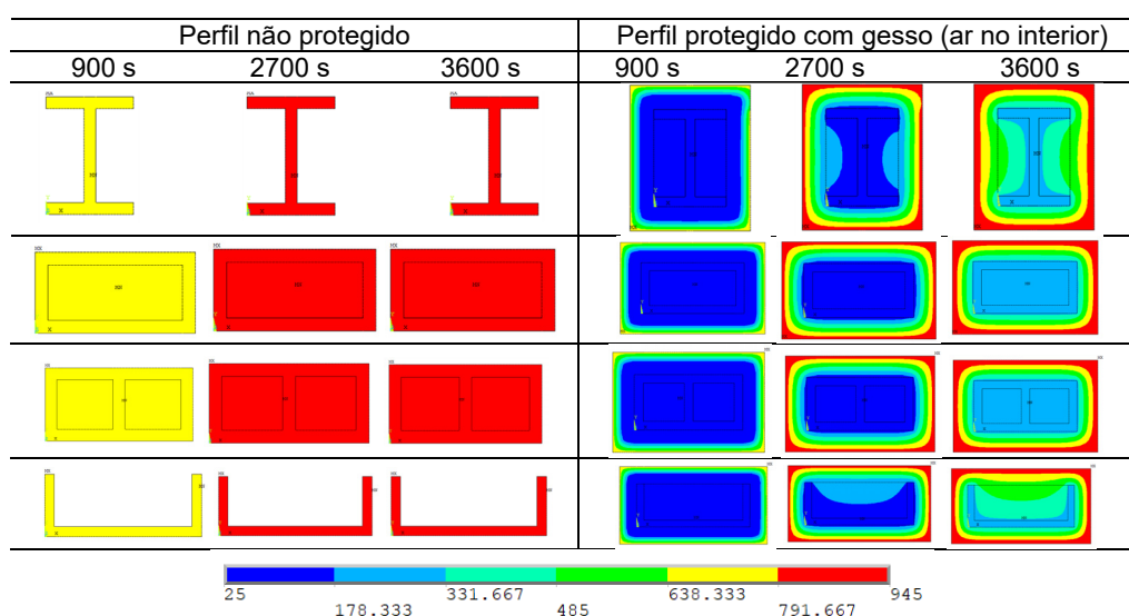
Figura 8: Temperaturas nos perfis não protegidos e com proteção em gesso tipo F.
