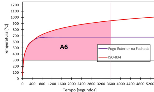
b) Área equivalente na curva ISO-834 para fogo exterior de fachada.
