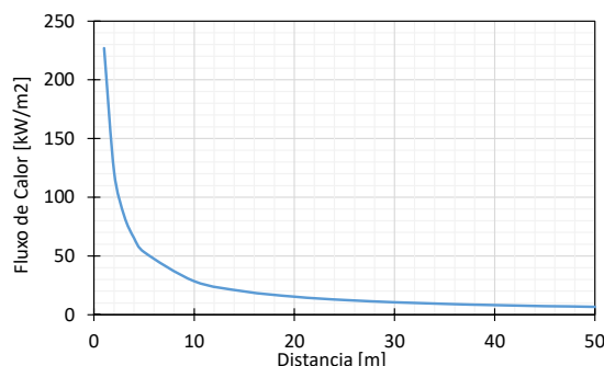
Figura 7: Fluxo de calor estacionário em função da distância da árvore ou arbusto a arder.
