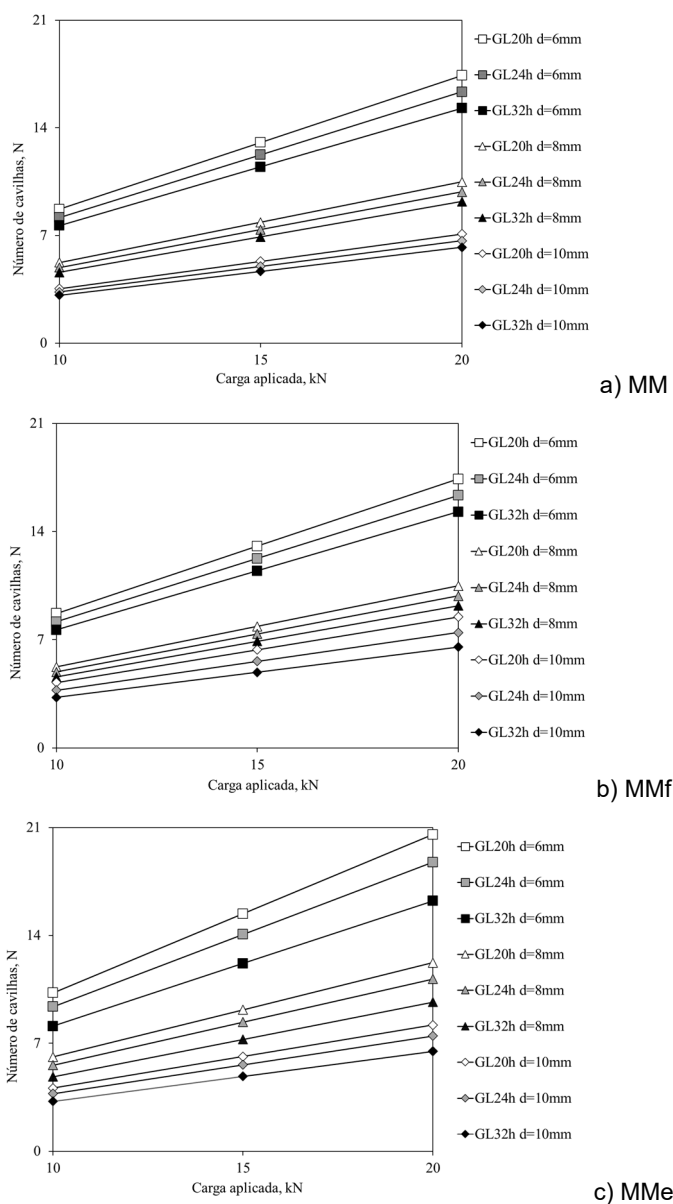
Figura 2: Número de cavilhas em função da carga aplicada. a) ligação madeira-madeira MM; b) ligação madeira-chapa fina MMf; c) ligação madeira-chapa espessa MMe
