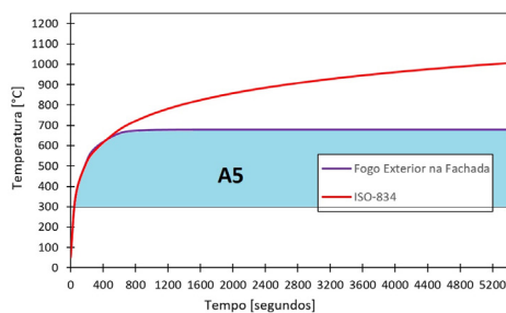
a) Área equivalente no fogo exterior de fachada.
