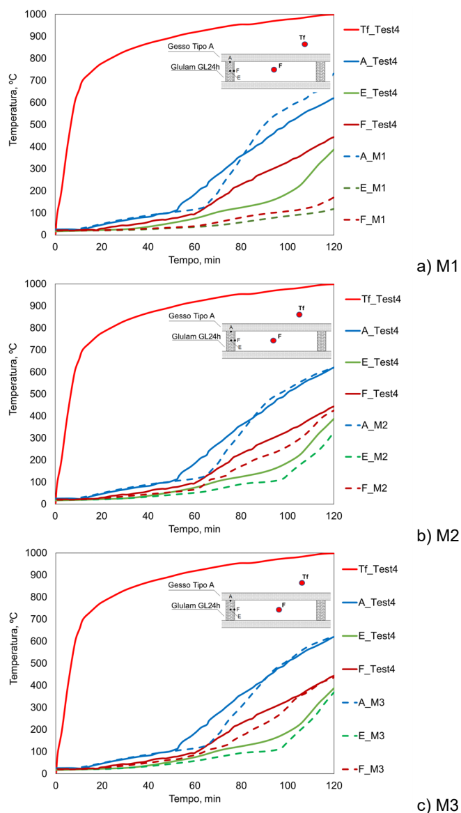
Figura 3: Resultados dos campos de temperatura.
