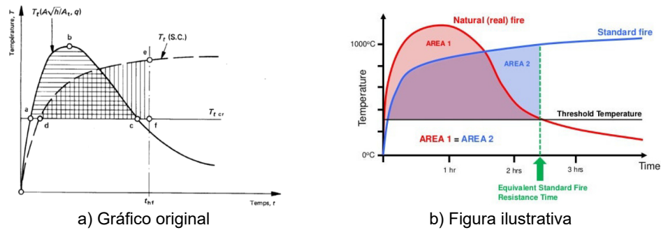
Figura 16: Método da área equivalente, para o cálculo do tempo equivalente de exposição da curva nominal ISO-834.
