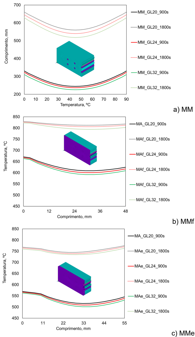
Figura 5: Temperatura na cavilha para dois instantes de tempo. a) ligação madeira-madeira MM; b) ligação madeira-chapa fina MMf; c) ligação madeira-chapa espessa MMe
