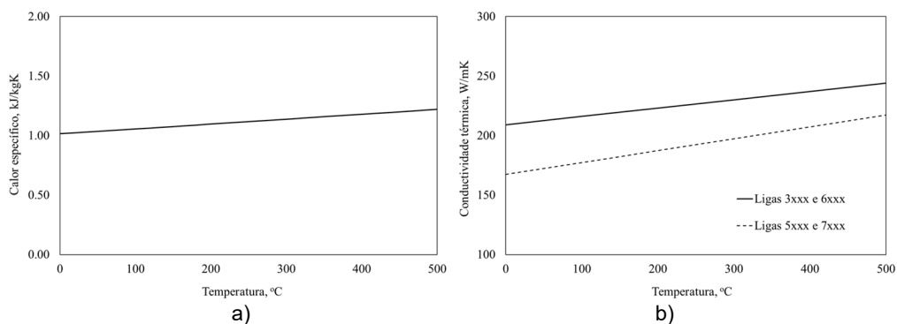
Figura 1: a) Calor específico e b) condutibilidade térmica do alumínio, função da temperatura
