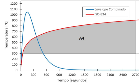
b) Área equivalente na curva ISO-834 para envelope de fogos em árvores e arbustos.
