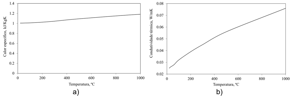
Figura 3: a) Calor específico e b) condutividade térmica do ar em função da temperatura
