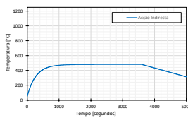
Figura 13: Cenário a) curva de acumulação de faúlhas.
