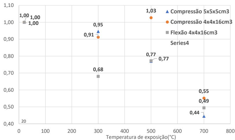
Figura 7 – Rácios das resistências em relação ao valor de referência (20°C).
