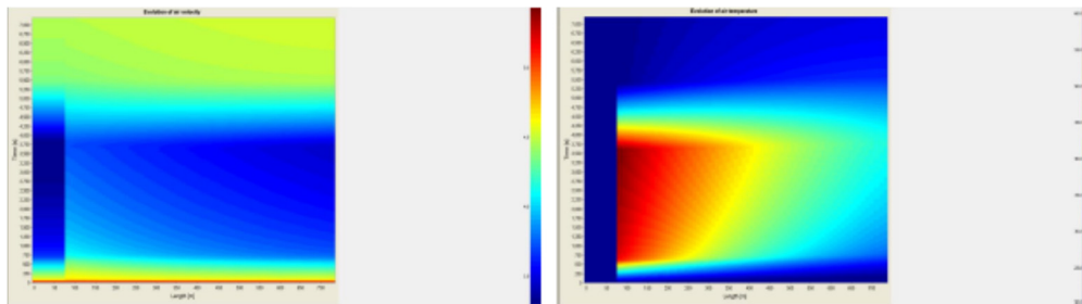
Figura 7 - Diagramas de Velocidade e Temperatura do ar/fumo
