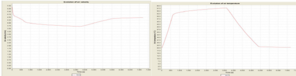
Figura 8 - Velocidade e Temperatura do ar/fumo na secção 60 m a jusante do foco
