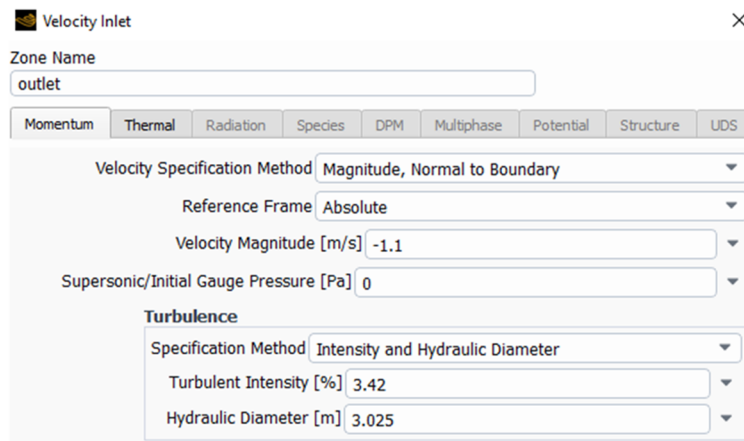
Figura 4: Definição da condição de fronteira de saída ( outlet )
