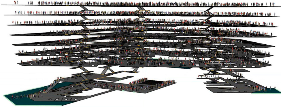
Figura 3: Imagem da simulação de evacuação com Pathfinder, mostrando-se uma visualização 3D no início da evacuação, com o edifício na máxima ocupação.
