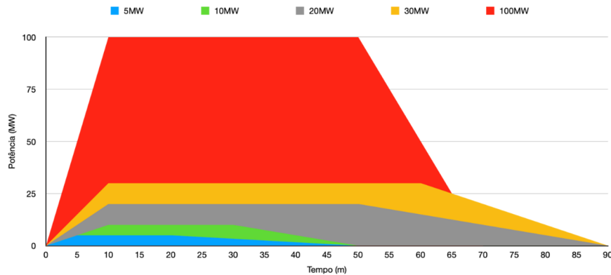
Figura 3 – Cenários de incêndio [7]
