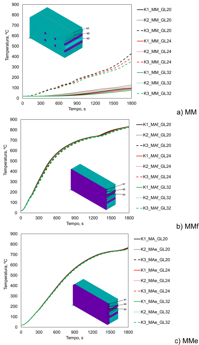
Figura 4: Evolução da temperatura. a) ligação madeira-madeira MM; b) ligação madeira-chapa fina MMf; c) ligação madeira-chapa espessa MMe
