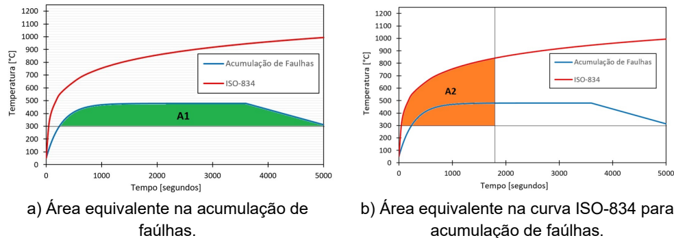
Figura 17: Método da área equivalente, para o cálculo do tempo equivalente de exposição da ação indireta do fogo florestal.
