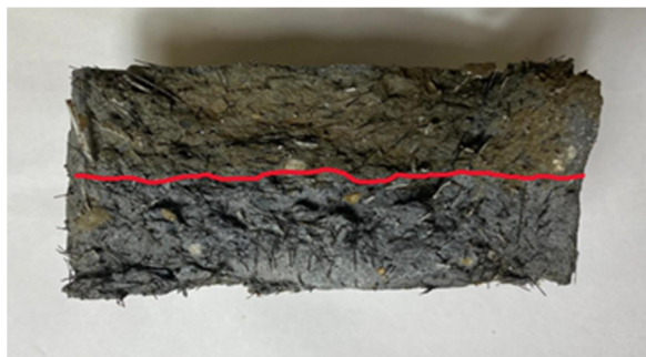
Figura 2 - Profundidade de penetração dos cloretos.
