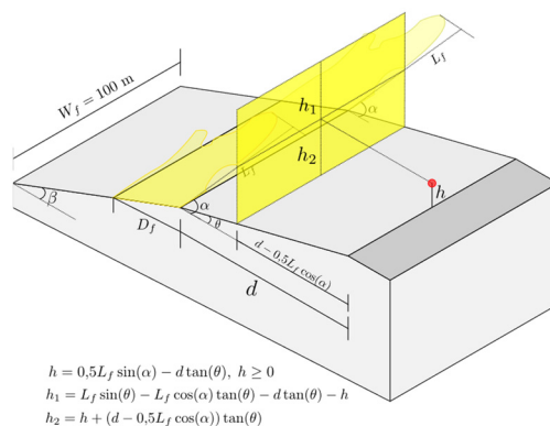
Figura 1: Modelo adotado na AS3959:2018 - plano com temperatura da chama
