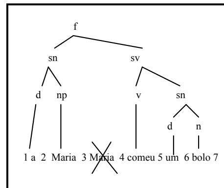
Fig. 3.3 Árvore sintáctica
