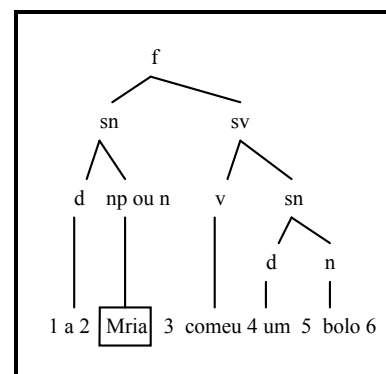
Fig. 3.5 Árvore sintáctica
