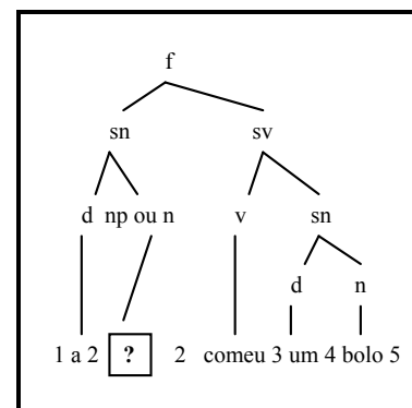
Fig. 3.4 Árvore sintáctica
