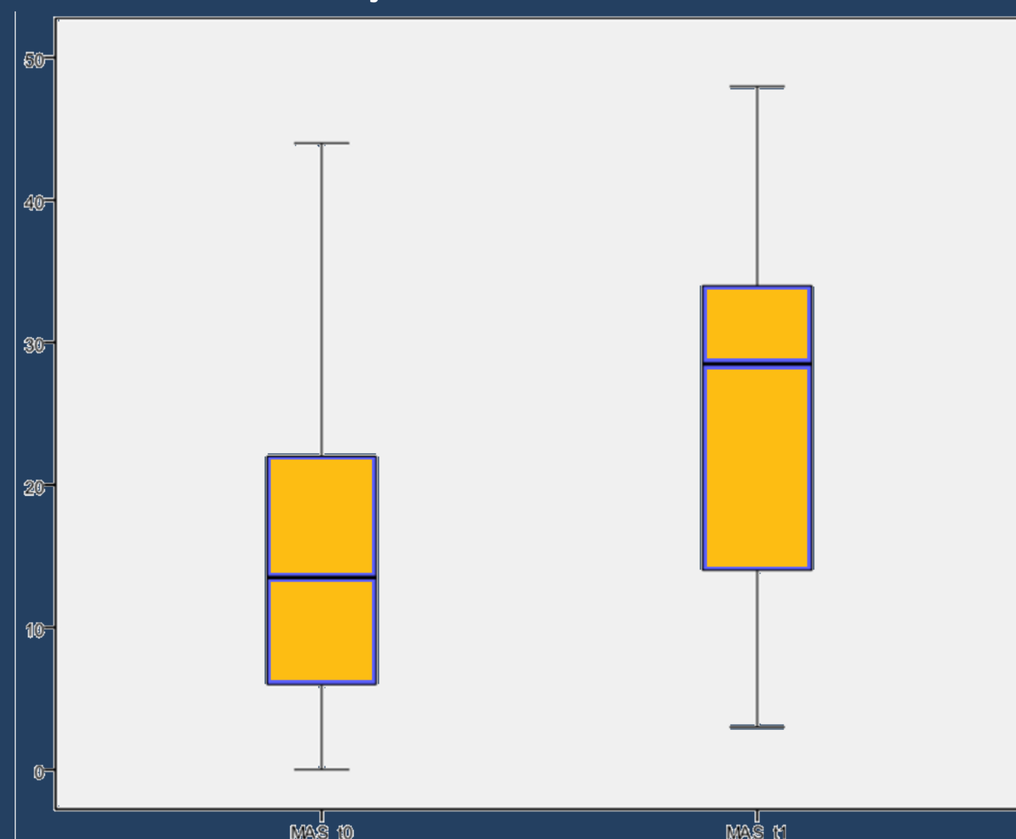
Gráfico 1– Pontuação Inicial e Final da MAS em t0 e t1.
