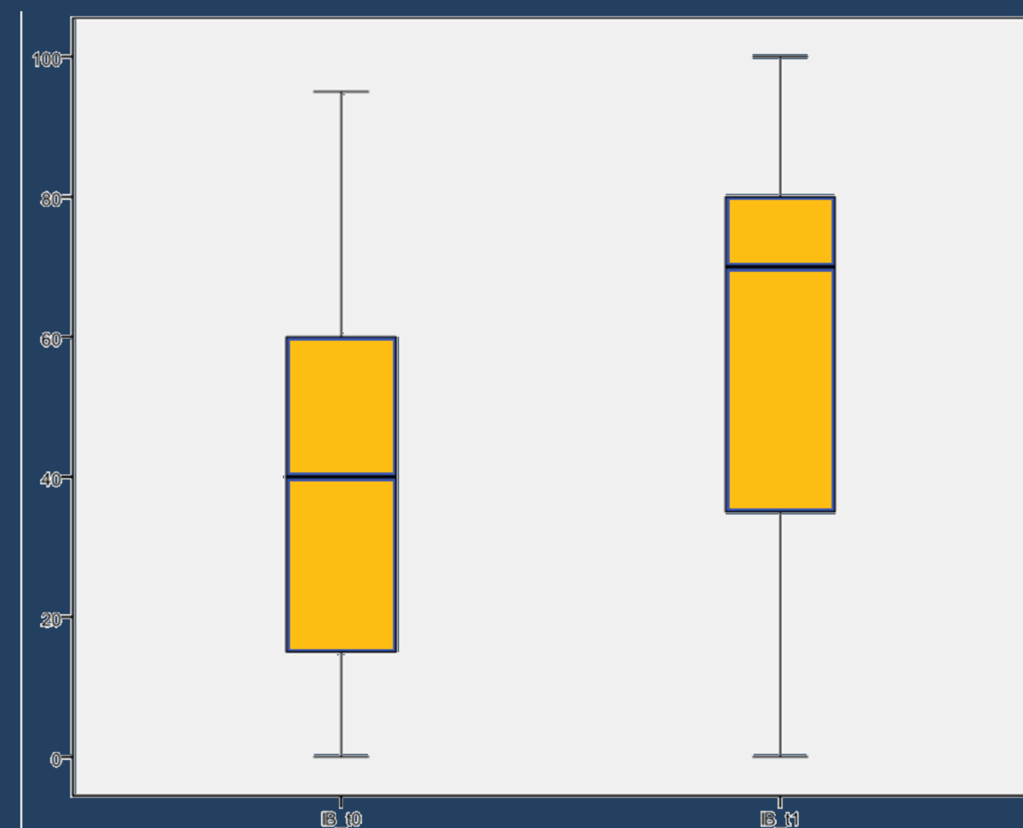
Gráfico 2– Pontuação Inicial e Final do IB em t0 e t1.
