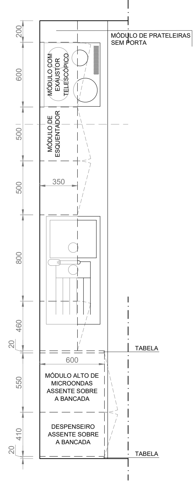
VISTA SUPERIOR - COTAGEM DOS MÓDULOS SUPERIORES
