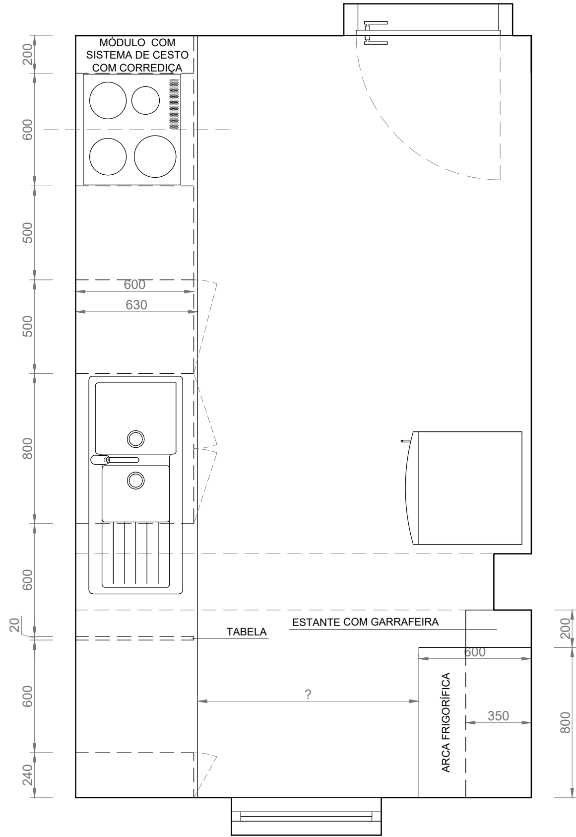
VISTA SUPERIOR - COTAGEM DOS MÓDULOS INFERIORES E MÓDULOS ALTOS
